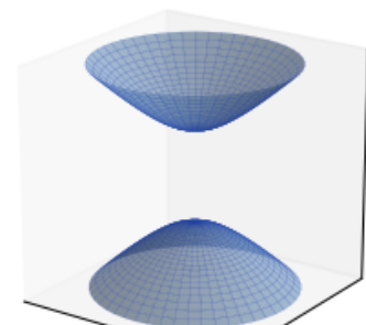
hyperboloïde à deux nappes x^2/a^2 + y^2/b^2 - z^2/c^2 = -1
