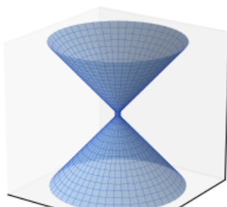
cône x^2/a^2 + y^2/b^2 - z^2/c^2 = 0
