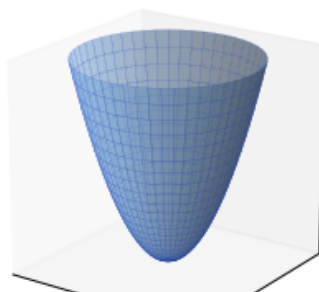
parabolôïde elliptique z = x^2/a^2 + y^2/b^2
