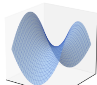
parabolôïde hyperbolique z = x^2/a^2 - y^2/b^2
