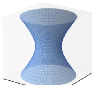
hyperboloïde à une nappe x^2/a^2 + y^2/b^2 - z^2/c^2 = 1
