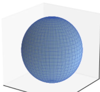
ellipsoïde x^2/a^2 + y^2/b^2 + z^2/c^2 = 1
